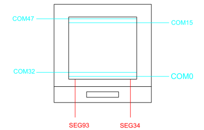
SEG&amp;COM Layout
