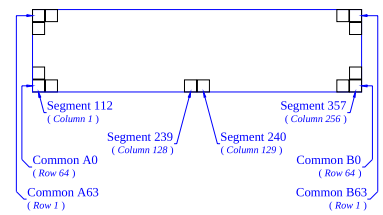
SEG & COM Layout
