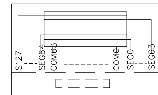
Com & Seg layout
